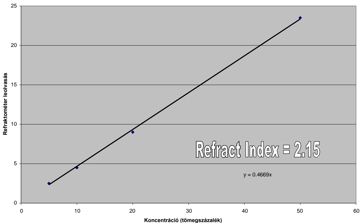
A VpCI-379 refraktométer görbéje
